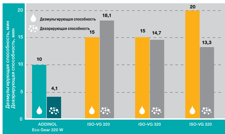
График 3. Деэмульгирующая и деаэрирующая способность синтетических трансмиссионных масел согласно стандартам DIN ISO 6614 (82 °C), DIN ISO 9120 (75 °C)
