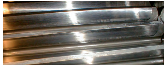
Ritzelwelle eines Zementmühlengetriebes Vor Umstellung auf ADDINOL Eco Gear bildete sich Graufleckigkeit am Zahnfuß. Nach Umölung wurde der Schadensverlauf gestoppt.
