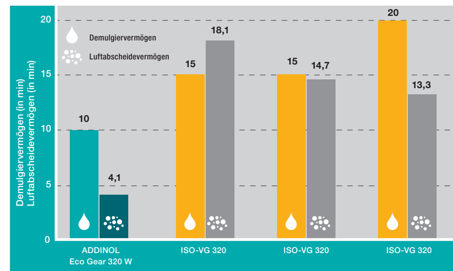
Grafik 3: Demulgier- und Luftabscheidungsvermögen synthetischer Getriebeöle nach DIN ISO 6614 (82 °C), DIN ISO 9120 (75 °C)
