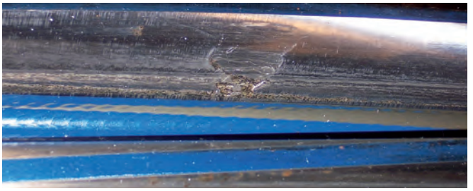
Ritzel eines Kalipressenantriebes, gehärtet-geschliffene Verzahnung Graufleckigkeit und Folgeschaden, Anrissstück wurde ausgeschliffen und das Ritzel weiterbetrieben.
